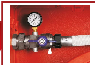
Valvola con manometro
